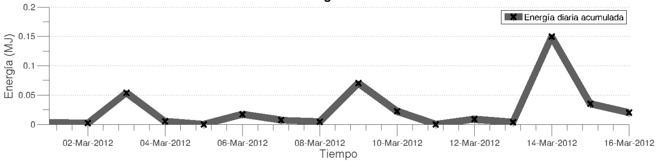
Sismicidad Dominante
