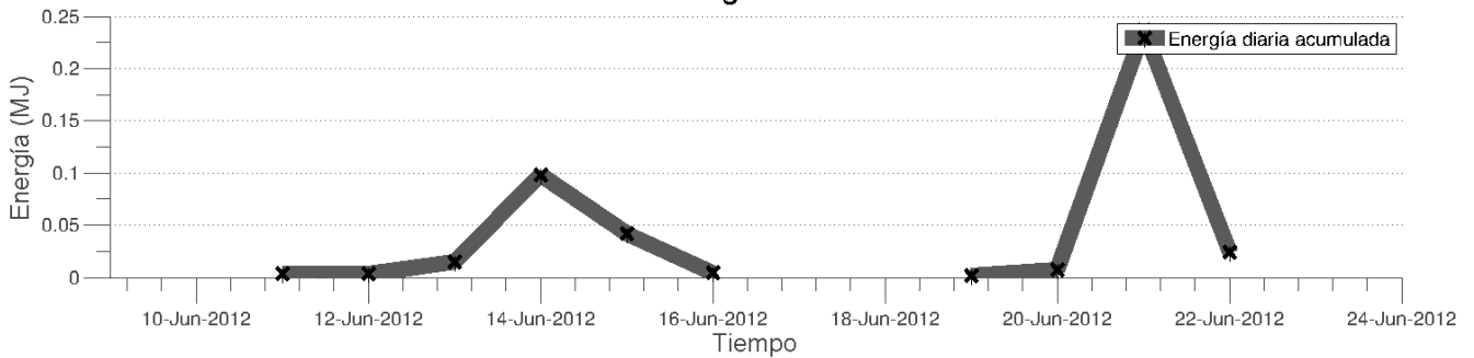
Sismicidad Dominante
