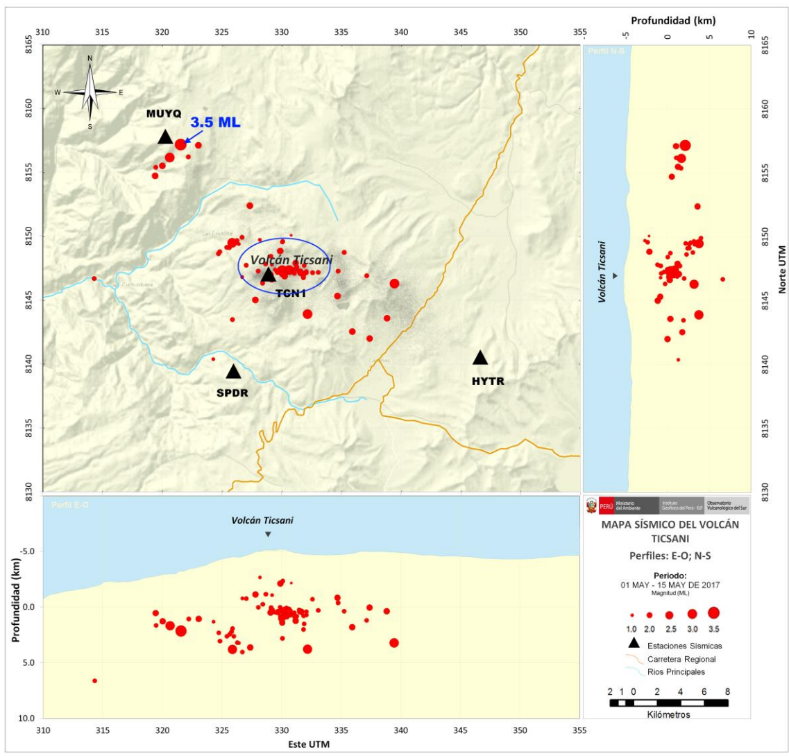
Figura 2.- Mapa de sismicidad para eventos de tipo fractura (VT) en el volcán Ticsani. Los círculos de color rojo representan los sismos ocurridos entre el 1 y 15 de mayo de 2017.
