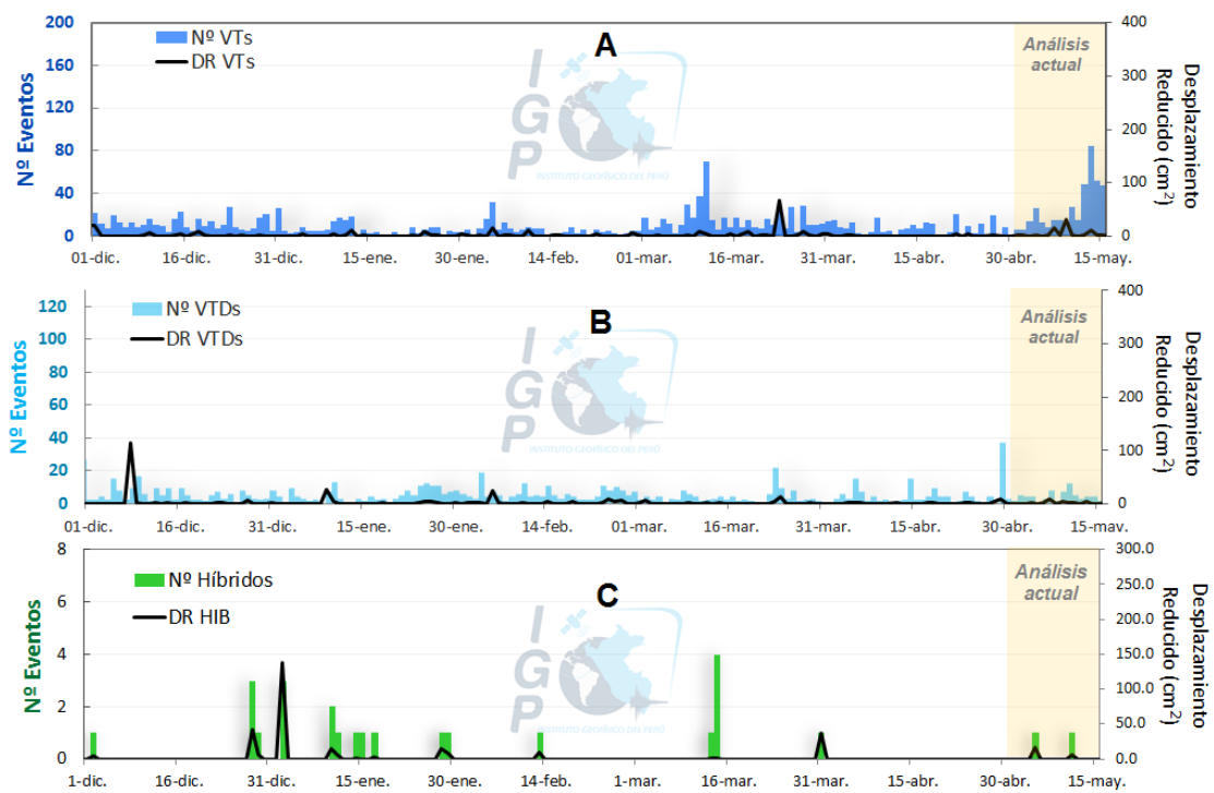
Figura 1.- Número de eventos registrados por la estación telemétrica TCN1 (barras de color) para los diferentes tipos de sismicidad analizada y el Desplazamiento Reducido DRmax. (Línea negra).
