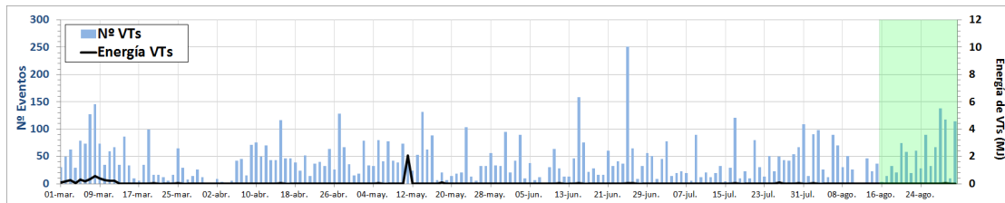
Figura 1.- Barras de color: tipo de eventos sísmicos registrados en el volcán Misti. Línea negra: energía sísmica calculada para cada tipo de evento sísmico. El sombreado verde representa el periodo de análisis del presente reporte.
